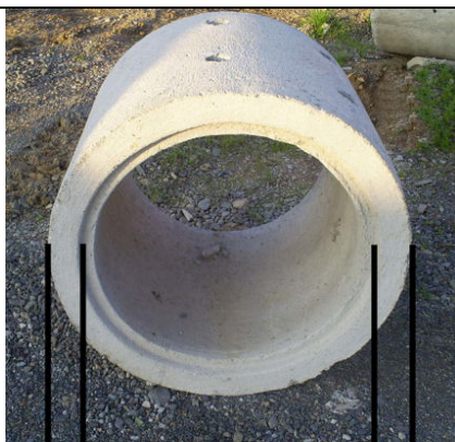
TUBO DE 0,80 X 0,50 – 330 Kls.
